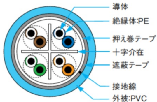
■構造図
