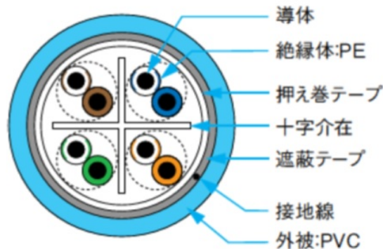
■構造図
