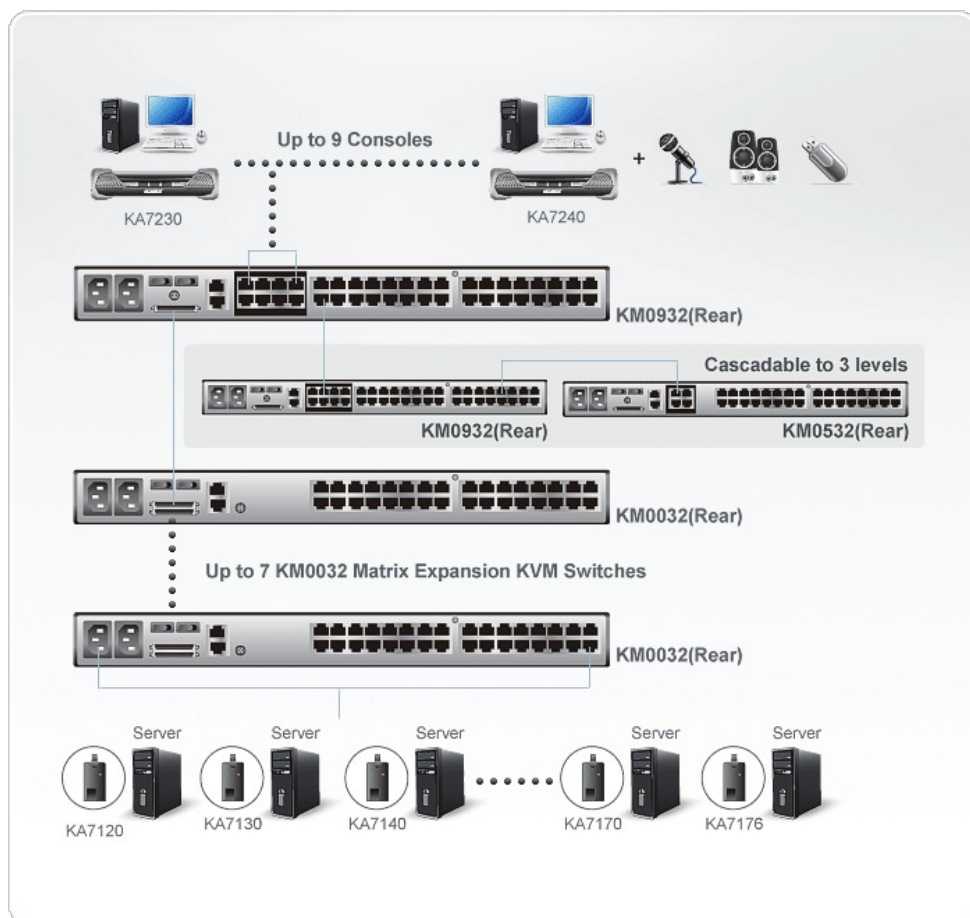
構成図
