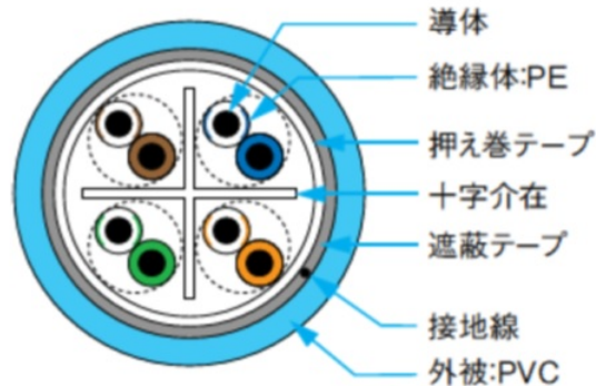
■構造図
