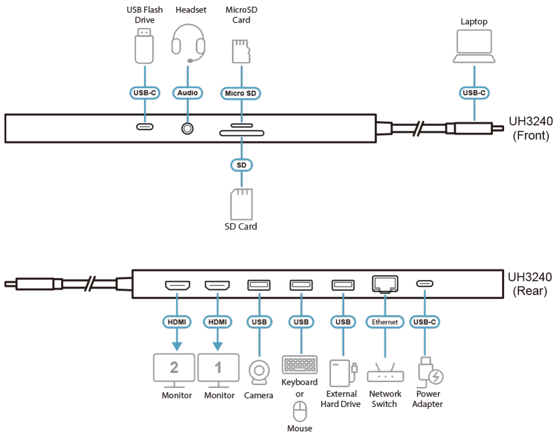
Diagrama
