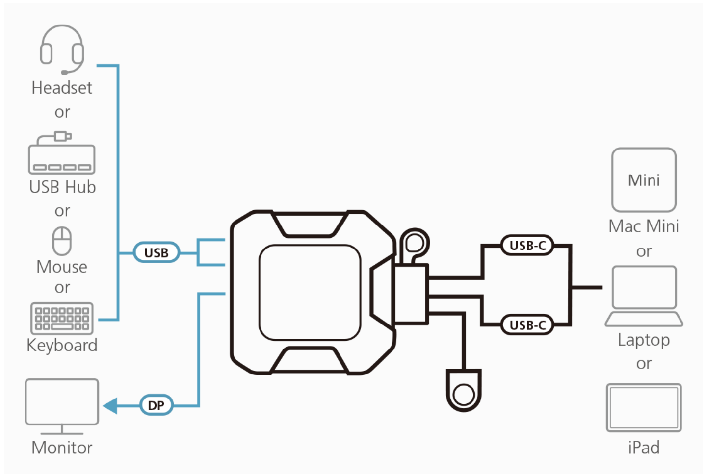
連線圖
