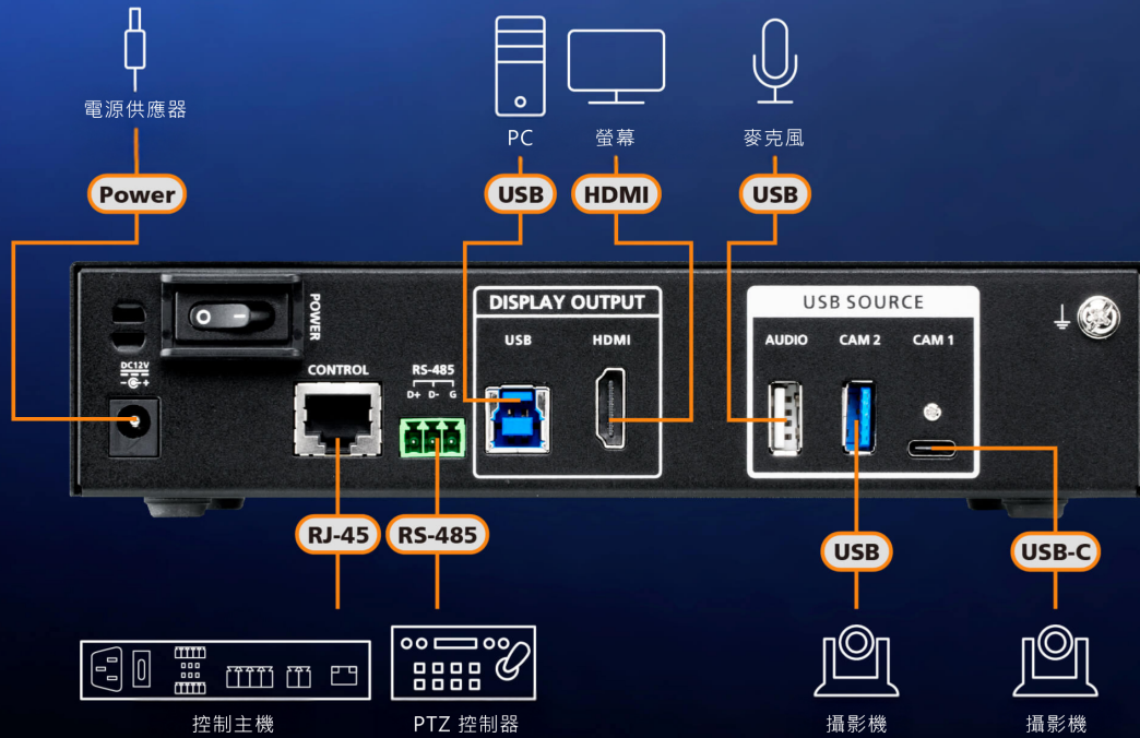
UC3310 背視圖
